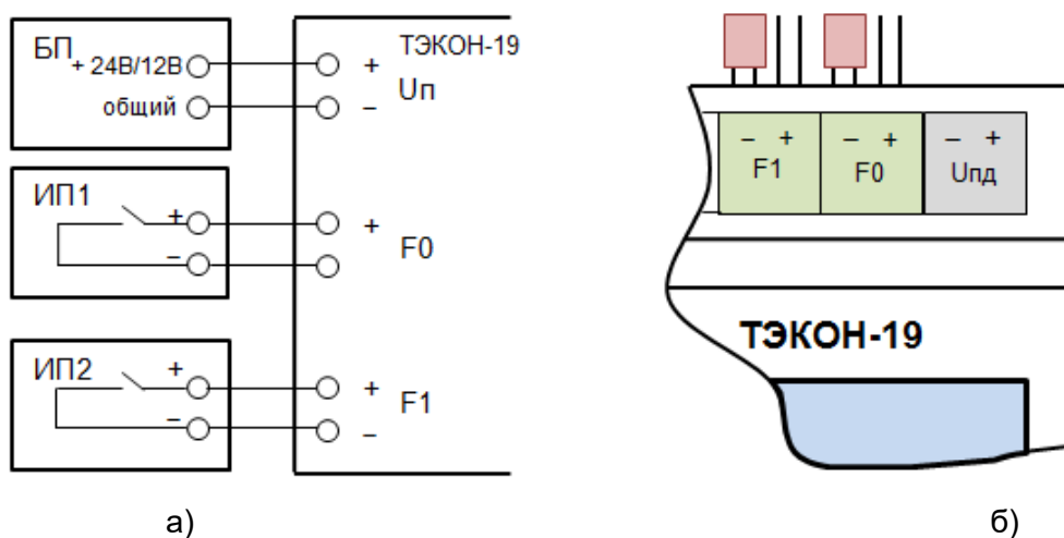
Рисунок 6 – Подключение ИП с числоимпульсным выходным сигналом типа сухой (пассивный) контакт с ограничением тока до 0,5 мА.
