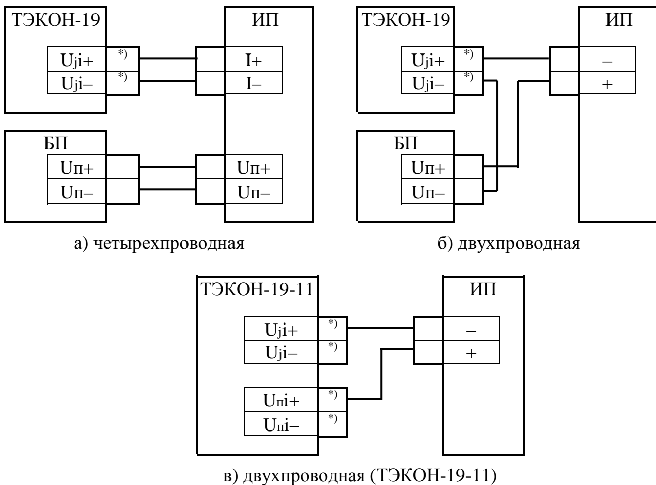
Рисунок 3.2 – Схемы подключения ИП с токовым выходом
