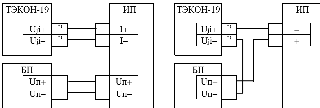
а) четырехпроводная
