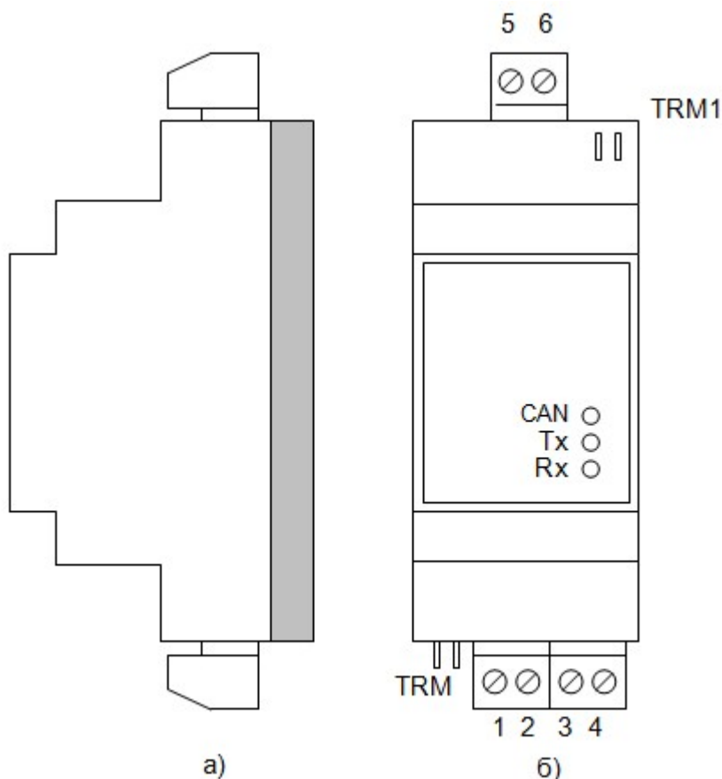
Рисунок 2.2. Внешний вид адаптера а) сбоку; б) с передней панели
