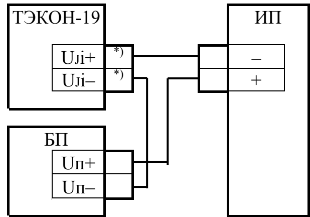
б) двухпроводная
