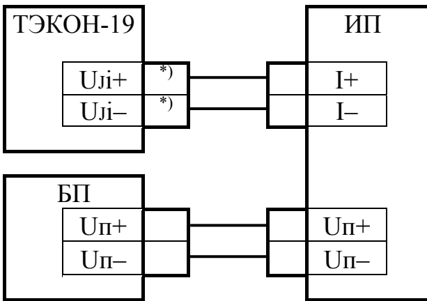
а) четырехпроводная
