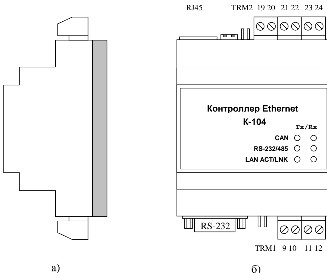
Рисунок 2.2 – Внешний вид Контроллера Ethernet К-104 а) сбоку; б) со стороны лицевой панели
